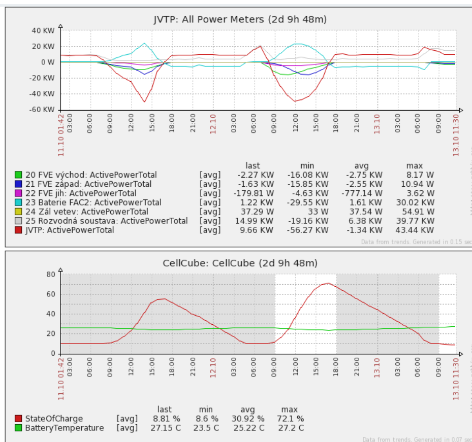
Obrázek 2: Power meters
